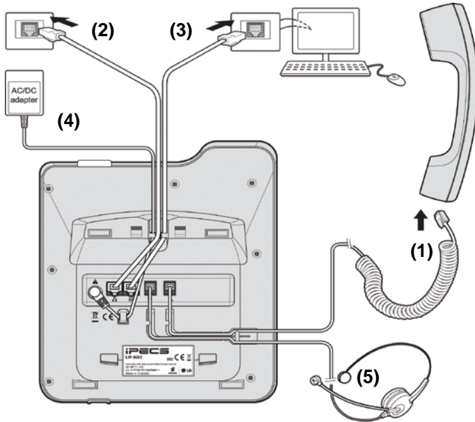
그림 8 LIP-9002 연결
