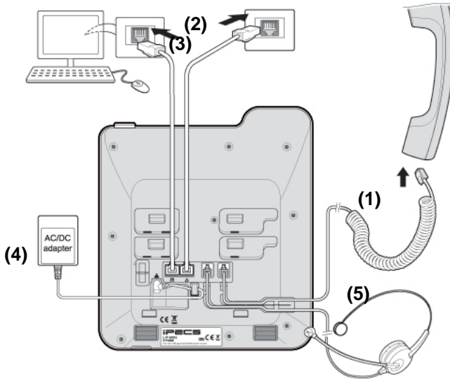
그림 9 LIP-9008/LIP-9008G 연결
