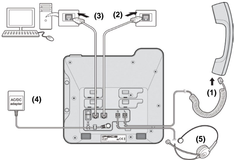
그림 10 LIP-9000 시리즈 연결
