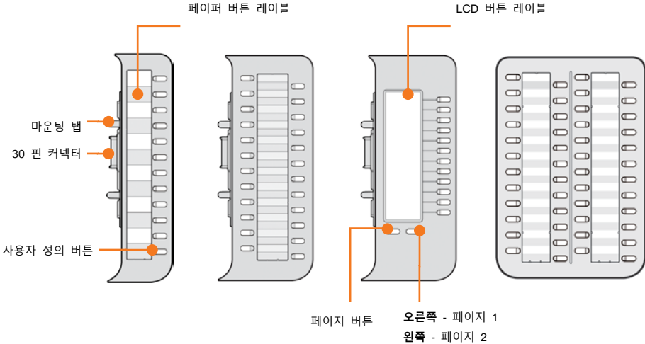
그림 2 LIP-9012 DSS, LIP-9024 DSS, LIP-9024 LSS, LIP-9048 DSS
