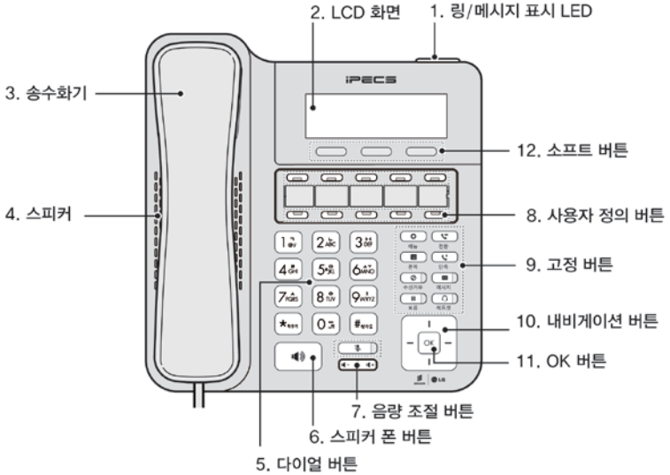
그림 4 LIP-9020 주요 부분 명칭
